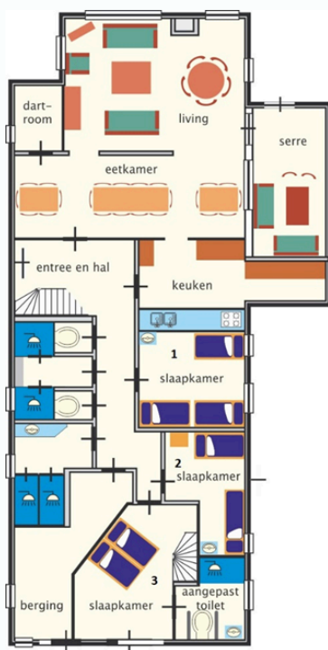
Erdgeschoss
